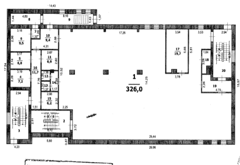
подвал 1:200
